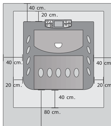
Slika 3. Minimalna udaljenost od predmeta
