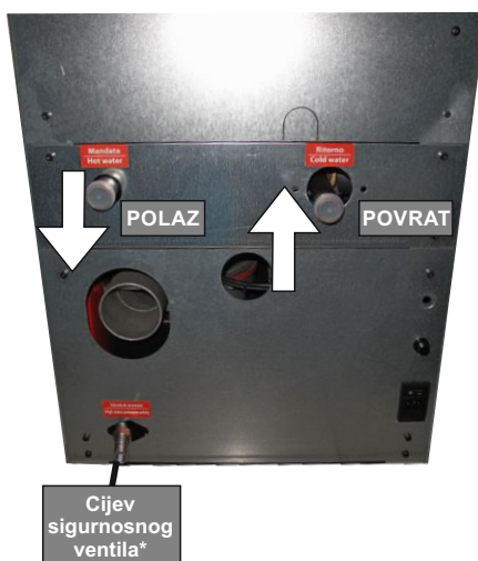
Slika 5. Polaz, povrat i cijev sigurnosnoga ventila
