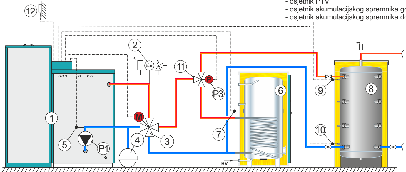
Shema 5. Konfiguracija PTV || AKU
