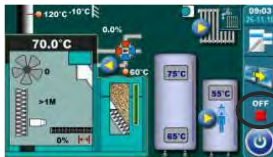
Oznaka stanja/ faze rada kotla
