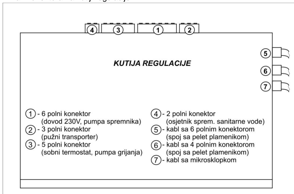
Slika: Prikaz konektora na kutiji regulacije
