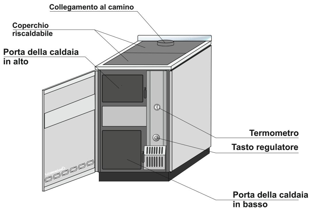
Foto 8. Componente generali
